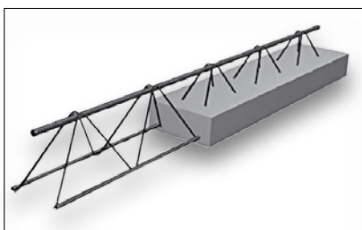
Sarruskarkass koorikpaneelis või kandetalas
