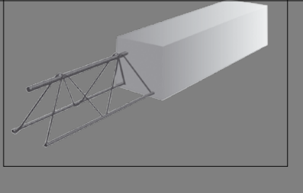
Tankorakenne filigran-paneelissa tai
