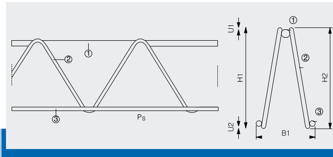
Raudoitustankorakenne filigran-paneelissa
