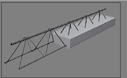
Tankorakenne filigran-paneelissa tai
