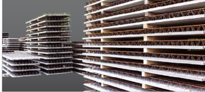
Raudoitustankorakenne filigran-paneelissa
